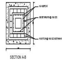
SECTION A-B
